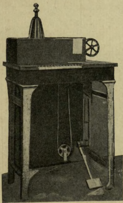
Австрійскій столъ съ клавишнымъ телеграфомъ.
