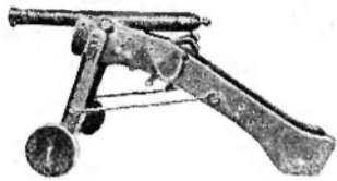
Первая горная пушка (1793 г.). хранится въ туринскомъ национ. музеѣ.
