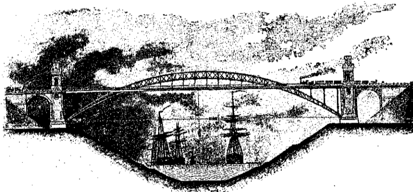
Какъ Германия готовилась къ войнѣ. Стверный каналъ. Поперечный разрѣзъ ложа канала и Большой мостъ у Грюненталя.
