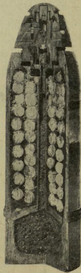
Разрѣзь шрапнели.
