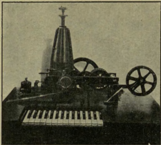
Австрійскій телеграфный аппаратъ съ буквенными клавишами.
